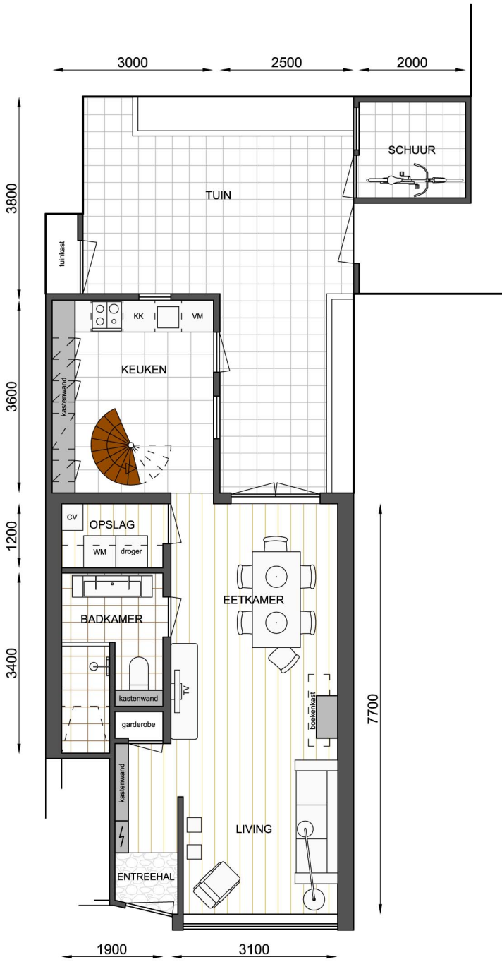
BEGANE GROND
